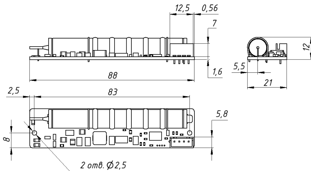
Чертеж 1. RadSens 1v6
